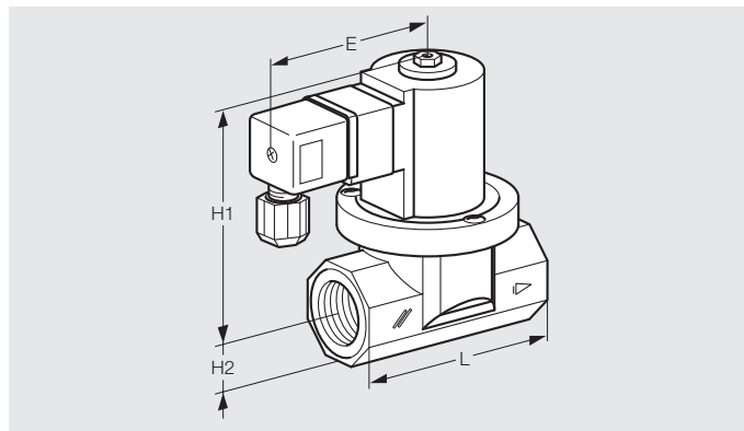
Datentabelle [mm]
